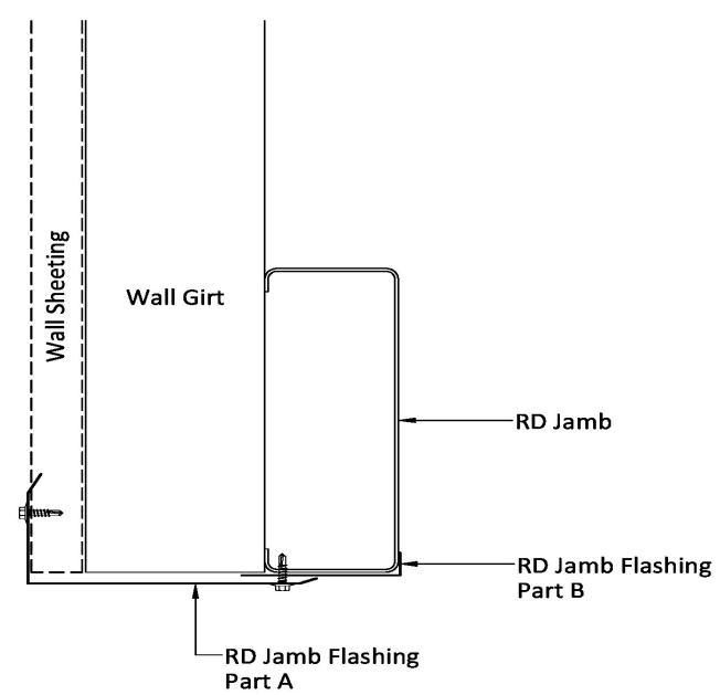
Roller Door Jamb Flashing - A-RDJAMB-I-A-0
